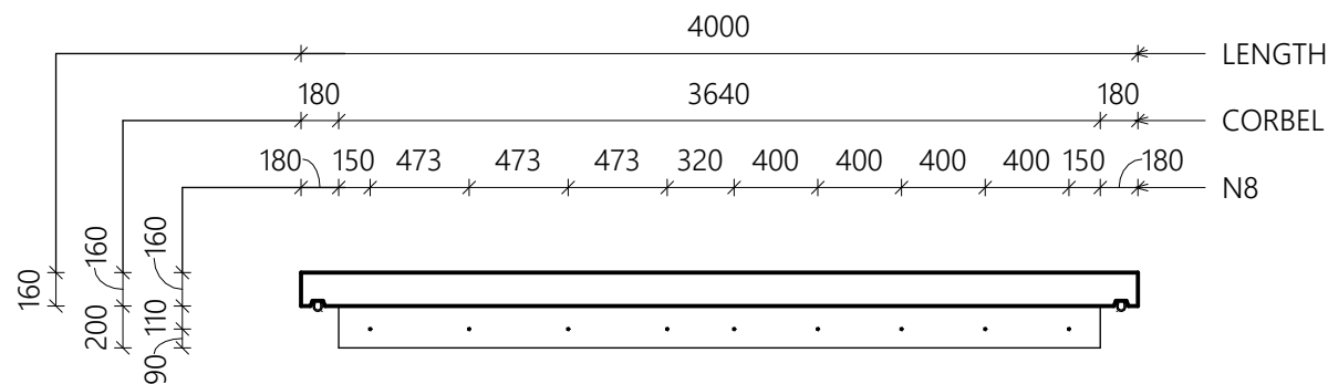
4 SECTION 1 : 40
