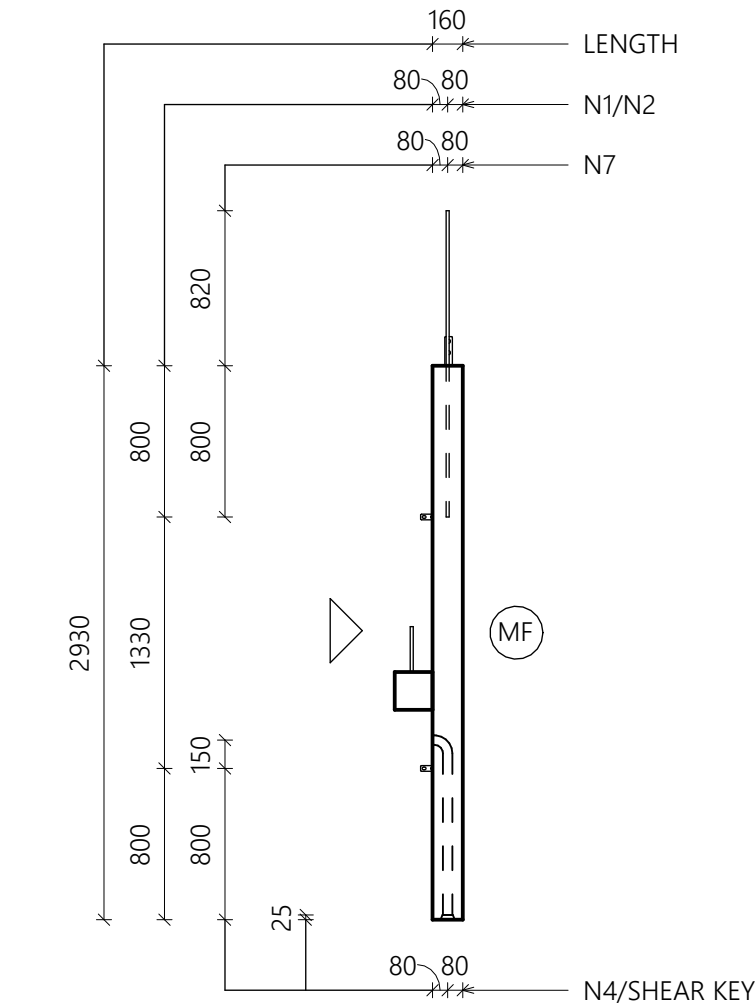
2 SECTION 1 : 40
