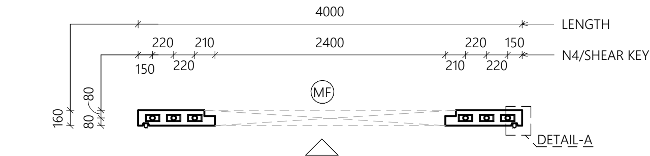
3 SECTION 1 : 40
